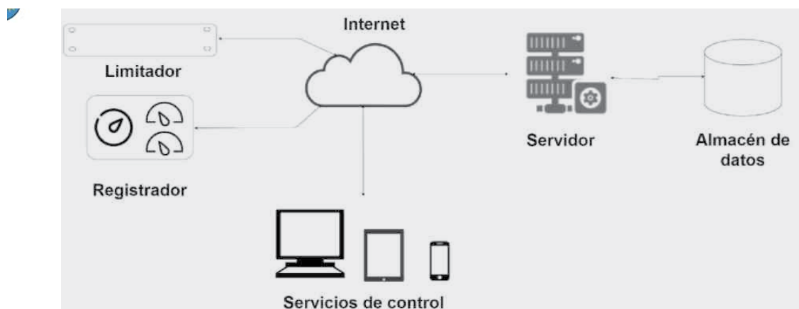
Arquitectura simplificada da plataforma de control de ruídos do Concello
